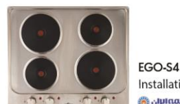
شعله کوچک: ۱۰۰۰ وات شعله متوسط: ۱۵۰۰ وات شعله بزرگ: ۲۰۰۰ وات EGO-S4 60 x 50 cm Installation Size: 565x470mm بیمه ایران E-G-O
